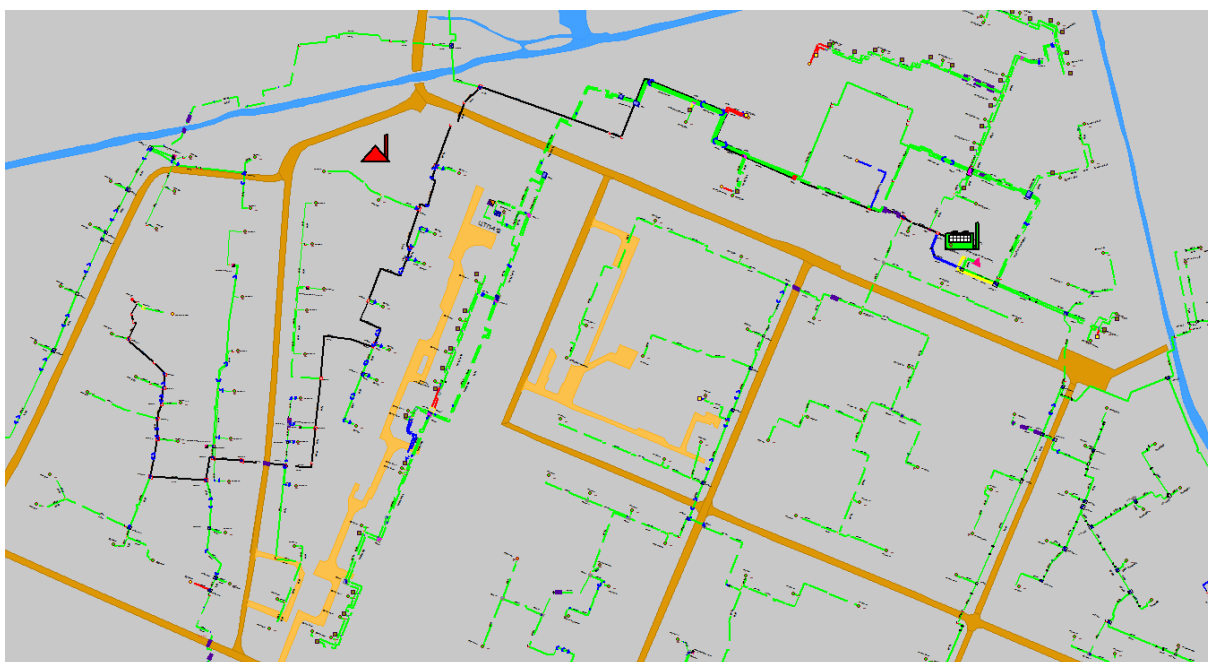
Рисунок 1.109 Результат гидравлического расчета - расчетный путь теплоносителя от котельной Премудрова, 12а до ПТ-Гвозд,8
