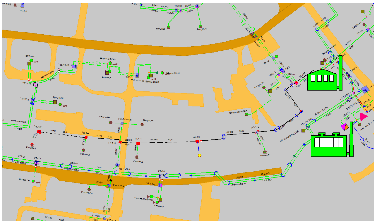
Рисунок 1.217 Результат гидравлического расчета - расчетный путь теплоносителя от котельной Батумская, 7-б до ПТ-Углова,1
