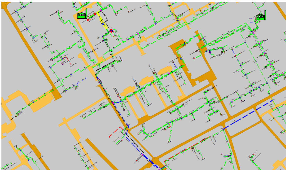
Рисунок 1.187 Результат гидравлического расчета - расчетный путь теплоносителя от котельной Баренца, 9а до ПТ-Иван.55а
