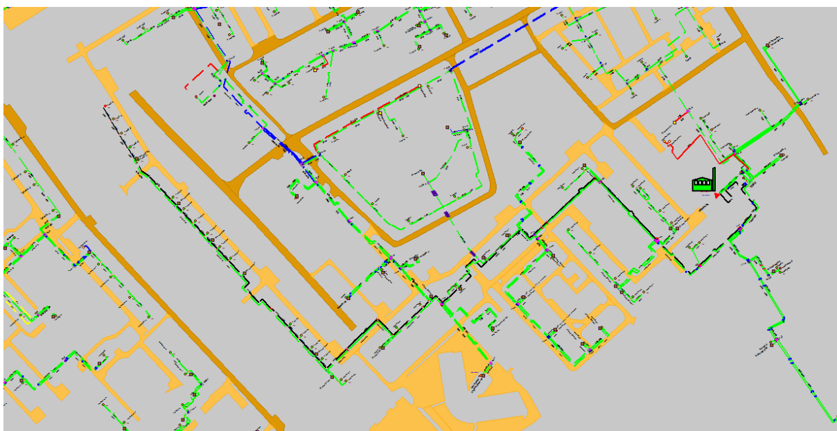
Рисунок 1.71 Результат гидравлического расчета - расчетный путь теплоносителя от котельной ул. Иванова, 14д до ПТ-Телег.3_э5
