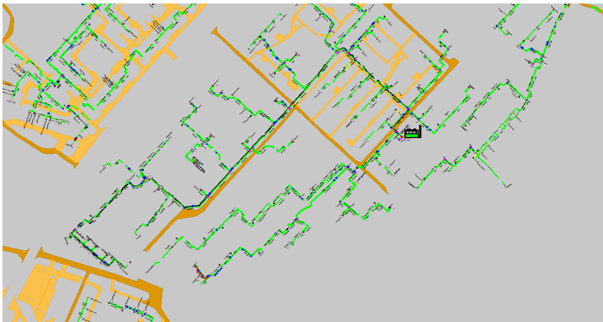
Рисунок 1.147 Результат гидравлического расчета - расчетный путь теплоносителя от котельной Военных комиссаров, 9 до ПТ-Гагар.пр,226 пристр
